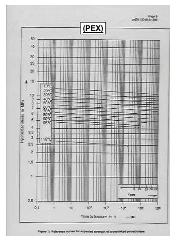
Las curvas de regresión de las tuberías Aqua Pipe tienen una forma lineal a elevadas temperaturas
